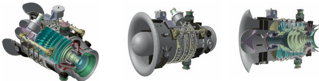
Рис. 2, 2а, 2б. Осевой компрессор низкого давления 6-ти ступенчатый, НПКГ «Зоря»—«Машпроект»
