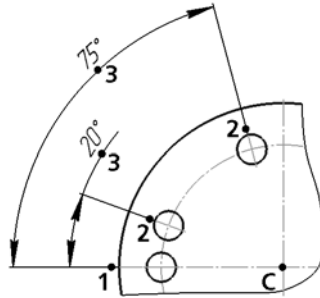
Рис. 3.3.39. Угловые размеры с ручным размещением размерной надписи; способ задания сторон угла — по двум отрезкам
