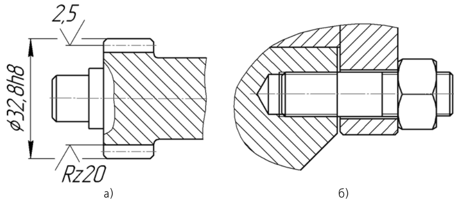
Рис. 3.5.37. Удаление части изображения: а) выносной линии размера, б) крепежного элемента (шпильки)
