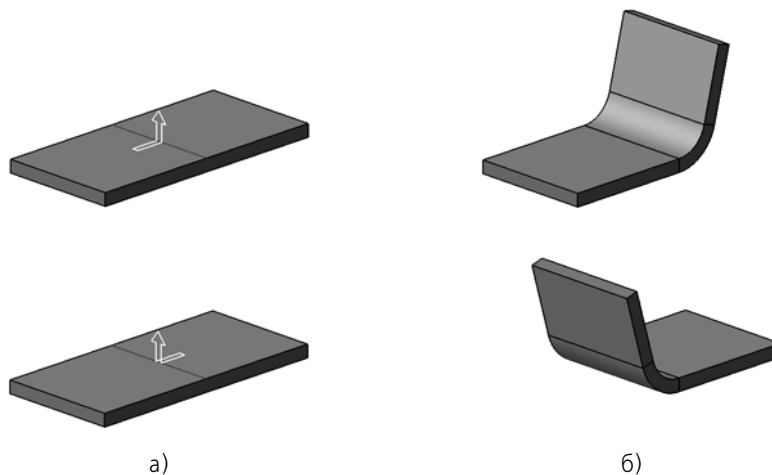
Рис. 2.4.51. Сгиб по линии: а) направление и неподвижная сторона, б) результат операции
