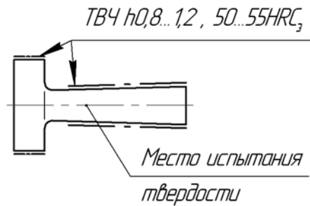
Рис. 3.3.55. Пример простановки линий-выносок
