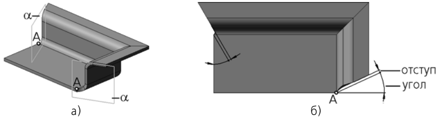
Рис. 2.4.80. Сгиб с замыканием в начале и конце: а) точка A и плоскость \alpha , б) вид сверху; отступ и угол
