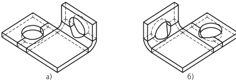
Рис. 2.4.88. Отверстия, построенные способом На глубину : а) вид детали сразу после создания отверстий, б) результат изменения состояния сгибов
