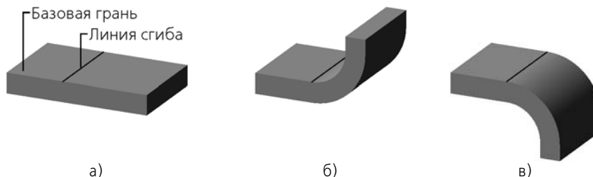
Рис. 2.4.27. Направление сгиба: а) базовая грань и линия сгиба, б) сгиб в прямом направлении, в) сгиб в обратном направлении
