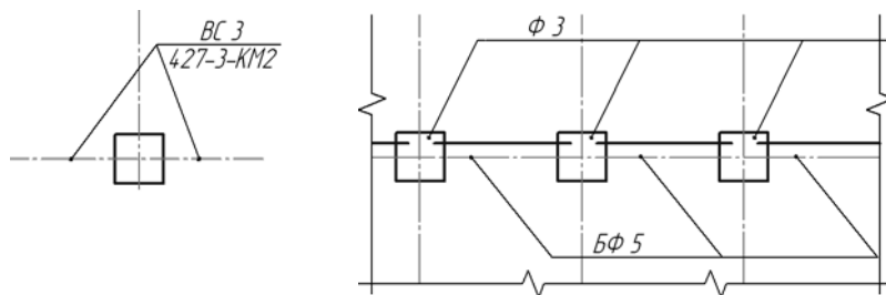
Рис. 3.3.106. Примеры марки/позиционного обозначения с линией-выноской
