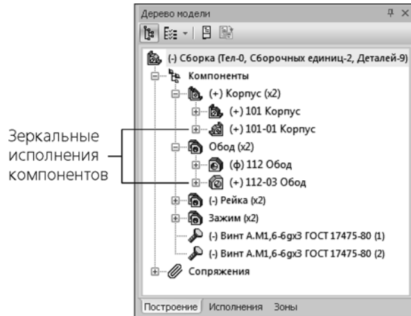
Рис. 2.11.8. Отображение зеркально отраженных компонентов в Дереве построения
