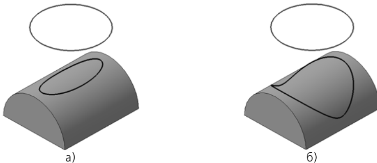
Рис. 2.5.54. Пример построения проекции линии эскиза на цилиндрическую поверхность: а) проецирование линии эскиза по нормали к поверхности; б) проецирование линии эскиза перпендикулярно плоскости эскиза
