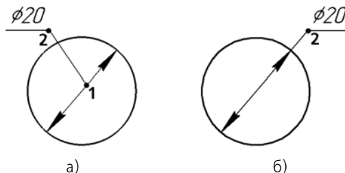
Рис. 3.3.24. Диаметральные размеры с надписью, размещенной на полке: а) линия-выноска не совпадает с размерной линией, б) линия-выноска совпадает с размерной линией
