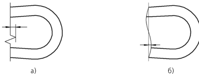
Рис. 3.6.18. Амплитуда: а) линии с изломом, б) волнистой линии (на рисунке также показана средняя линия)
