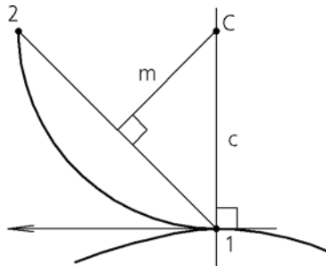
Рис. 2.5.19. Определение центральной точки дуги и радиуса
