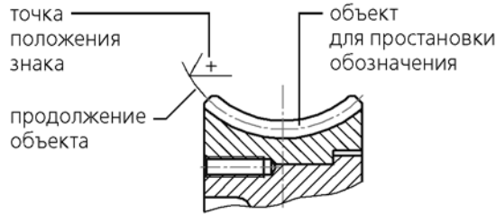
Рис. 3.3.50. Простановка обозначения шероховатости на продолжении объекта
