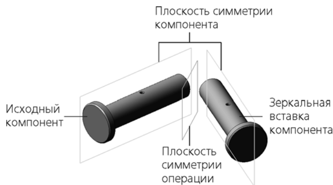
Рис. 2.11.6. Зеркальная вставка компонента, обладающего симметрией
