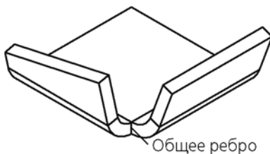
Рис. 2.4.58. Смежные сгибы
