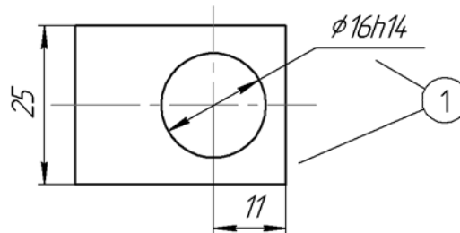
Рис. 3.3.68. Простановка обозначения изменения
