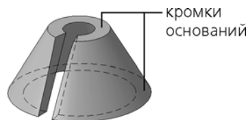
Рис. 2.4.14. Кромки оснований обечайки
