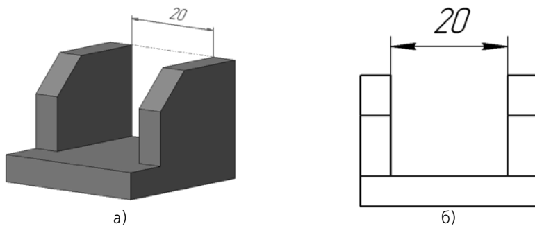
Рис. 3.7.12. Линейный размер в модели (а) и соответствующий ему проекционный размер в ассоциативном виде (б)
