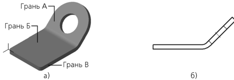
Рис. 2.4.102. Листовое тело: а) в проекции Изометрия XYZ , б) главный вид
