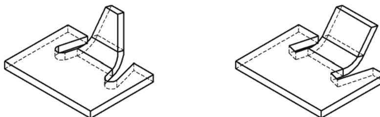
Рис. 2.4.46. Освобождение сгиба при отличном от нуля угле на сгибе
