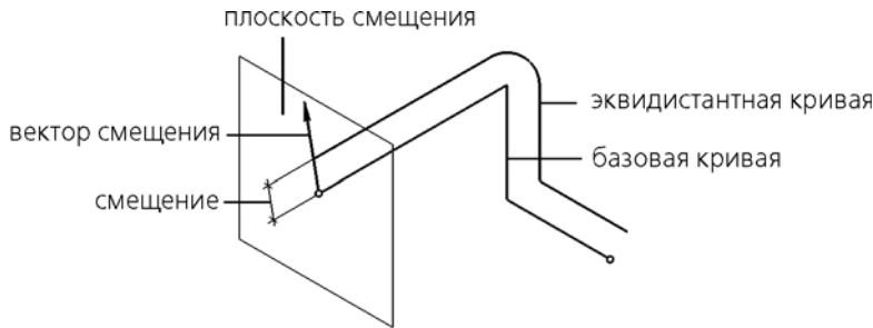
Рис. 2.5.44. Построение эквидистантной кривой способом Смещение по направлению от вершины
