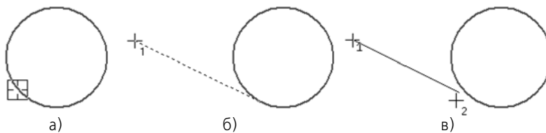
Рис. 3.2.57. Построение первого отрезка линии касательно к другому объекту: а) указание объекта, б) указание начальной точки отрезка, в) указание конечной точки отрезка
