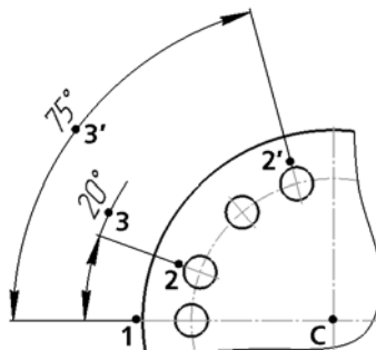
Рис. 3.3.41. Простановка угловых размеров от общей базы; способ задания сторон угла — по двум отрезкам
