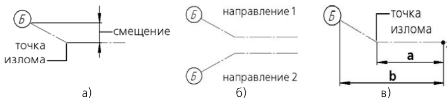
Рис. 3.3.127. Параметры выступа координационной оси: а) смещение, б) направление, в) смещение излома
