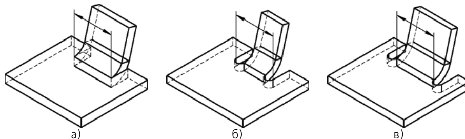
Рис. 2.4.45. Расположение освобождений: а) ширина сгиба без освобождений, б) освобождения включены в ширину сгиба, в) освобождения не включены в ширину сгиба
