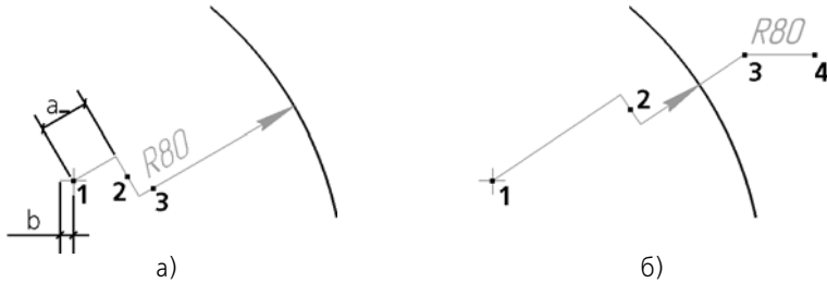
Рис. 3.3.32. Характерные точки размера с надписью, размещенной: а) вручную, б) на полке
