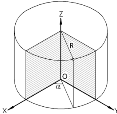
Рис. 2.5.12. Построение точки по цилиндрическим координатам; XYZ – система координат точки
