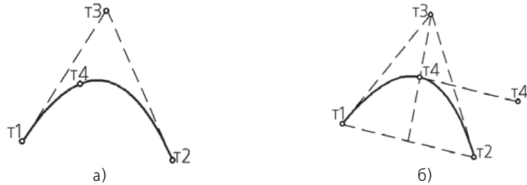
Рис. 3.2.54. Определение положения точки т4 : а) точка указана внутри треугольника при активном переключателе коэффициент; б) построение точки на медиане
