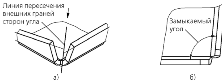
Рис. 2.4.61. Измерение зазора: а) определение положения плоскости измерения, б) проекция детали на плоскость измерения (вид по стрелке); замыкаемый угол
