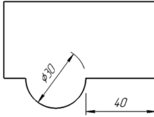
Рис. 3.3.10. Пример простановки линейного и диаметрального размеров с зазором
