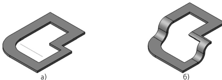
Рис. 2.4.53. Использование вспомогательной оси в качестве линии сгиба подсечки: а) расположение оси, б) результат построения
