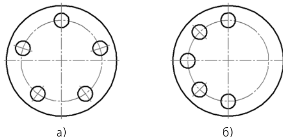
Рис. 3.5.19. Режим копирования: а) вдоль всей окружности, б) с угловым шагом 45°
