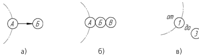
Рис. 3.3.132. Элементы дополнительных обозначений круговой оси: а) указатель ориентации, б) марка, в) текст
