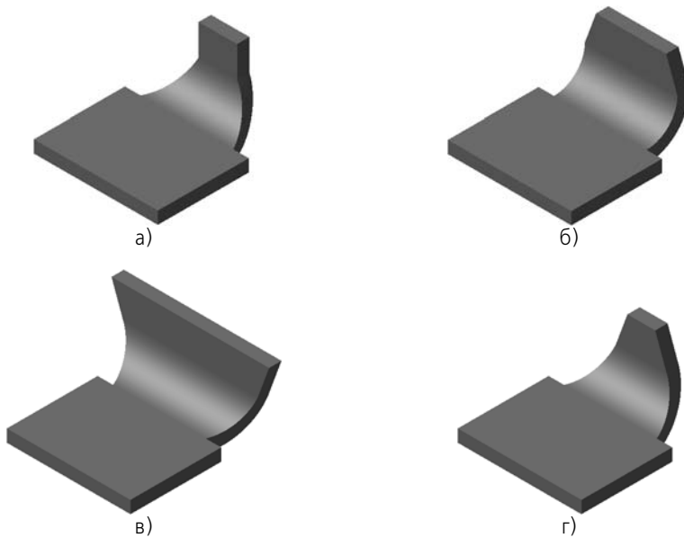
Рис. 2.4.43. Управление боковыми сторонами сгиба: а) углы на сгибе, б) уклон боковых сторон продолжения сгиба, в), г) углы на сгибе и уклон боковых сторон продолжения
