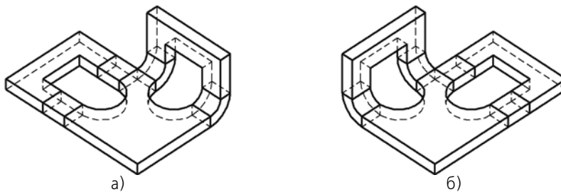
Рис. 2.4.91. Вырезы, построенные способом По толщине : а) вид детали сразу после создания вырезов, б) результат изменения состояния сгибов
