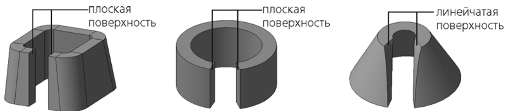
Рис. 2.4.17. Построение кромок стыка способом Перпендикулярно поверхности листа
