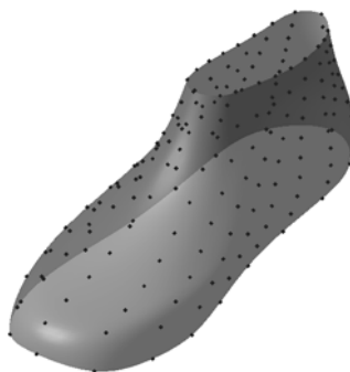
Рис. 2.6.11. Поверхность по сети точек
