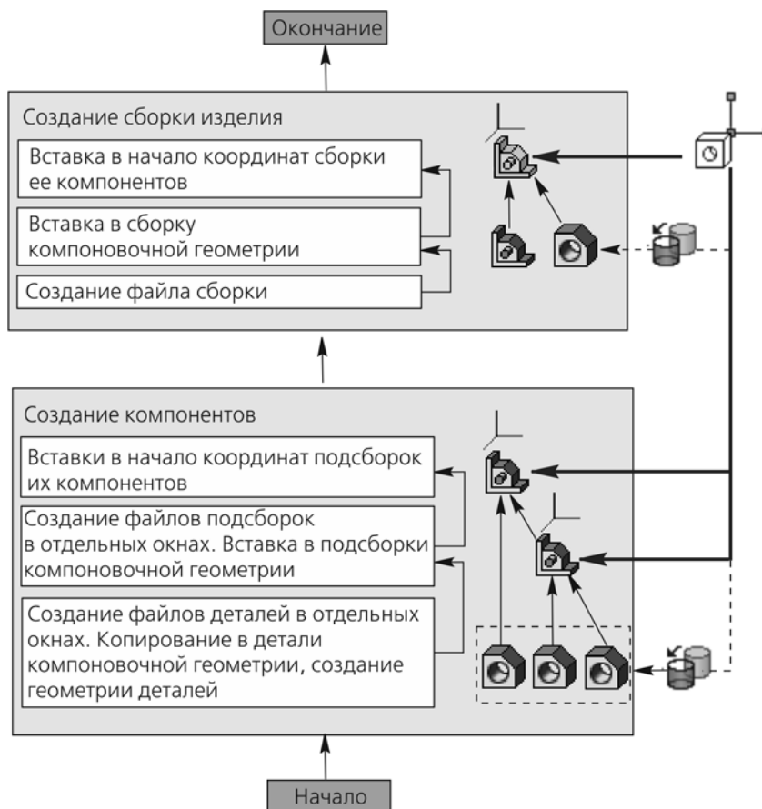
Схема проектирования снизу вверх с предварительной компоновкой
