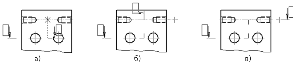
Рис. 3.3.73. Создание линии ступенчатого разреза:
