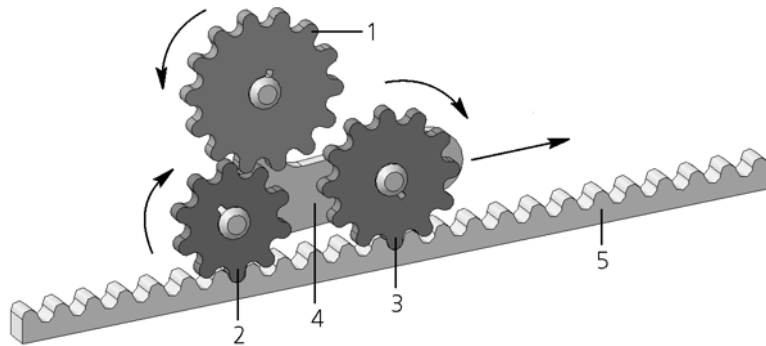
Рис. 2.11.15. Пример связи перемещений между деталями
