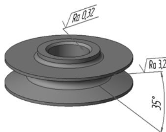
Рис. 2.9.20. Пример простановки обозначения шероховатости
