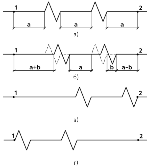
Рис. 3.3.99. Смещение изломов
