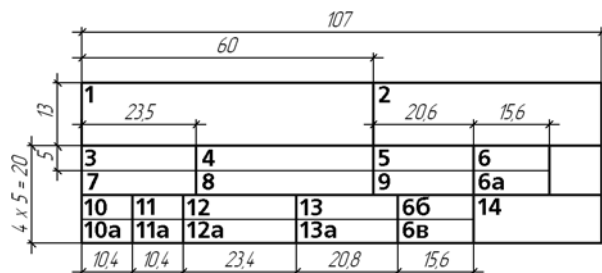
Рис. 11.2.15. Структура и размеры дополнительного штампа
