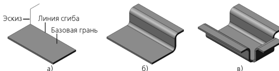
Рис. 2.4.74. Сгиб по эскизу: а) эскиз сгиба, б) сгиб вдоль одного ребра, в) сгиб вдоль нескольких ребер
