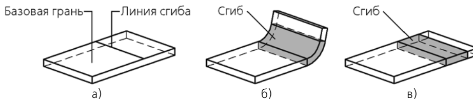
Рис. 2.4.31. Построение сгиба: а) базовая грань и линия сгиба, б) согнутый сгиб, в) разогнутый сгиб
