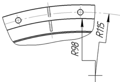
Рис. 3.3.29. Радиальные размеры с изломом
