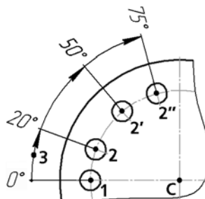
Рис. 3.3.43. Простановка угловых размеров с общей размерной линией; способ задания сторон угла — по трем точкам
