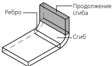
Рис. 2.4.36. Продолжение сгиба вдоль ребра
