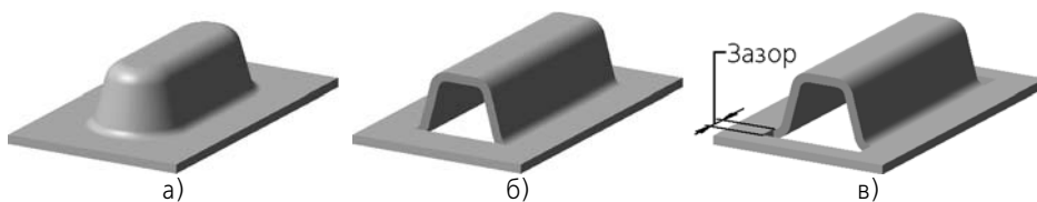
Рис. 2.4.114. Типы обработки концов буртика
