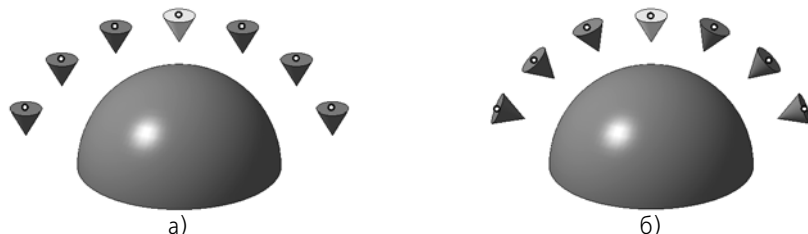
Рис. 2.7.38. Пример расположения экземпляров массива (базовый экземпляр выделен цветом): а) с сохранением исходной ориентации; б) с ориентацией по сферической грани
