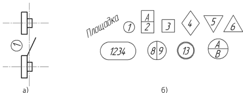
Рис. 3.3.104. Марка/позиционное обозначение без линии-выноски а) пример использования, б) типы формы обозначения
