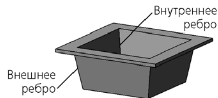
Рис. 2.4.108. Внутренние и внешние боковые ребра штамповки
