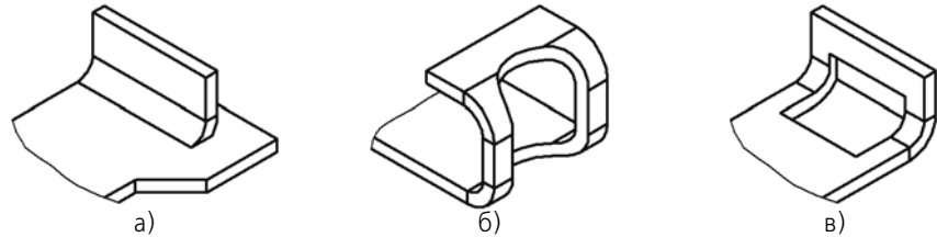
Рис. 2.4.98. Примеры листовых элементов, делающих невозможным разгибание сгиба: а) пластина, б) отверстие, в) вырез
