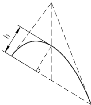
Рис. 10. Высота конической кривой
