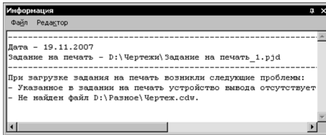
Рис. 8.5.3. Информационное окно
