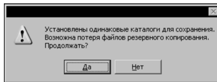
Рис. 9.1.5.
