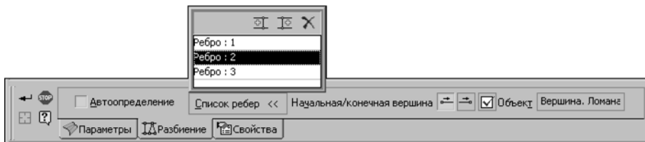
Рис. 2.6.22. Вкладка Разбиение
