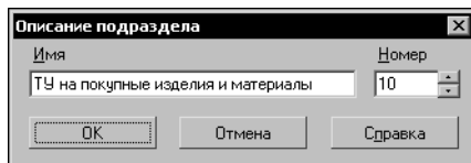
Рис. 6.4.5. Описание подраздела
