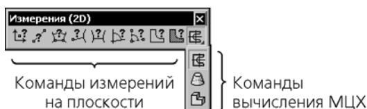
Рис. 3.9.1. Панель Измерения(2D)
