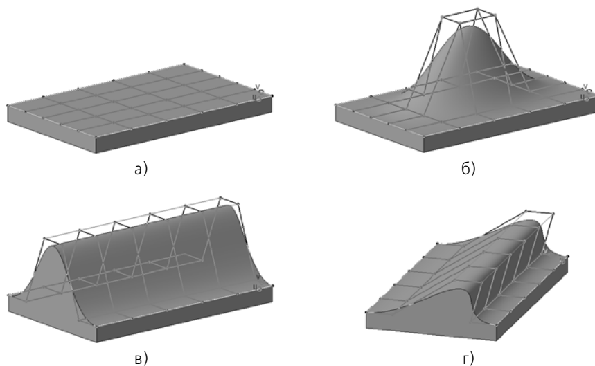
Рис. 2.6.38. Перемещение полюсов:
