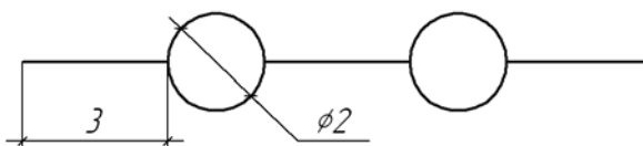
Рис. 11.1.17. Размеры элементов
