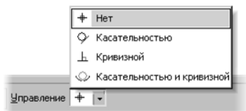
Рис. 2.5.24. Список Управление
