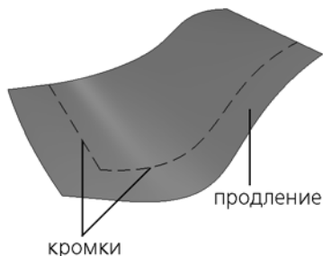
Рис. 2.6.34. Продление грани
