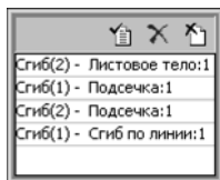
Рис. 2.4.95.
