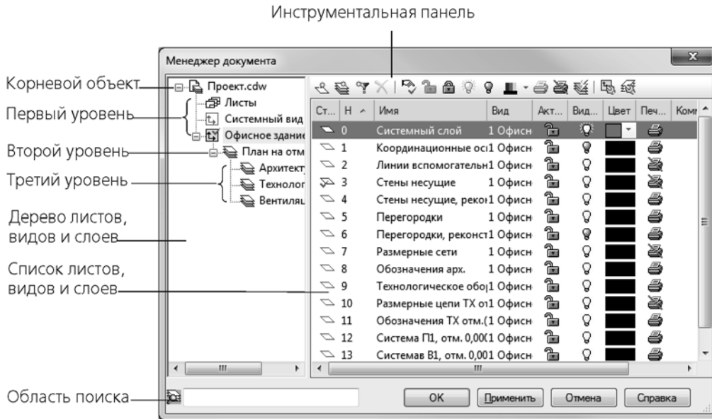
Рис. 3.6.20. Менеджер документа
