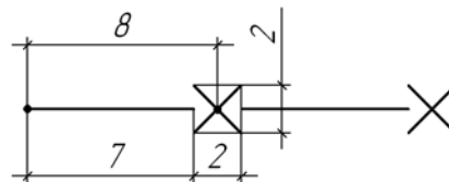
Рис. 11.1.21. Размеры элементов
