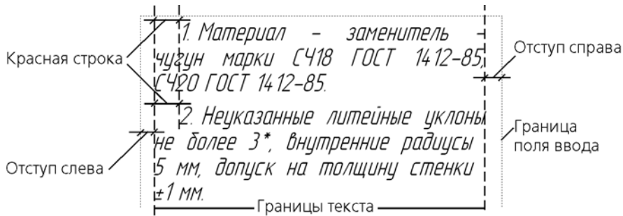
Рис. 11.1.40. Параметры абзаца
