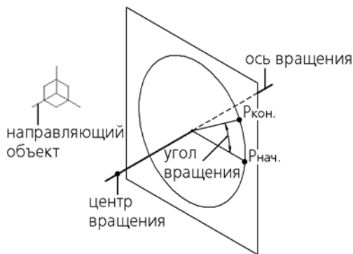
Рис. 2.6.48. Вращение полюса
