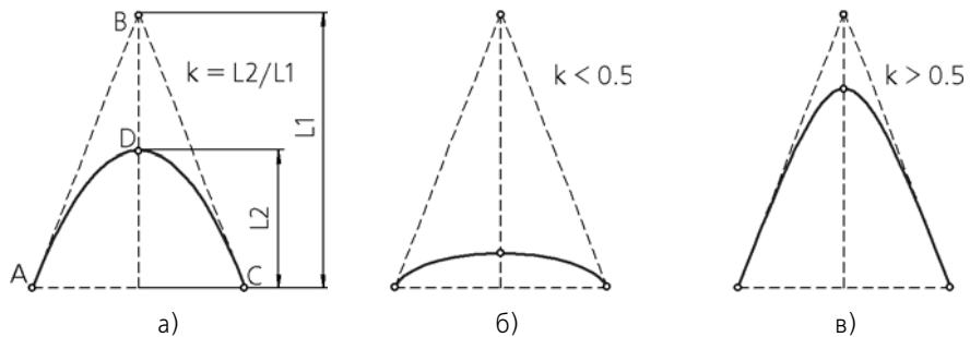
Рис. 9. Зависимость типа конической кривой от величины коэффициента: а) парабола; б) эллипс; в) гипербола
