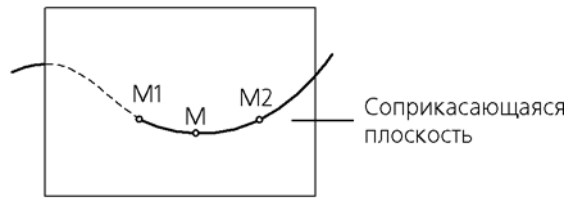
Рис. 6. Соприкасающаяся плоскость
