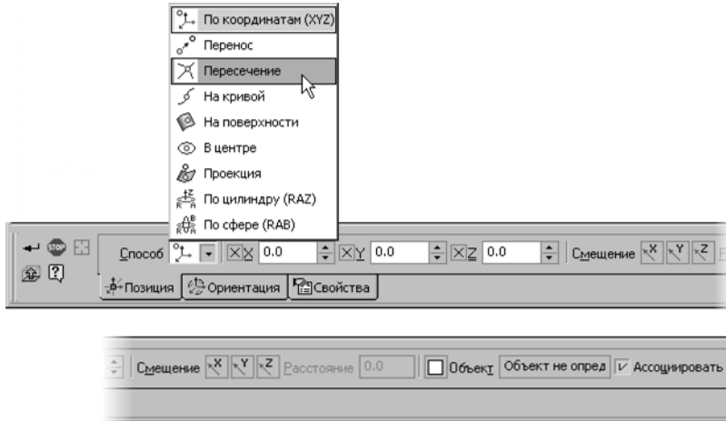
Рис. 2.8.8. Вкладка Позиция
