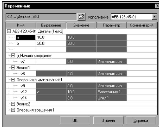
Рис. 7.1.8. Диалог Переменные
