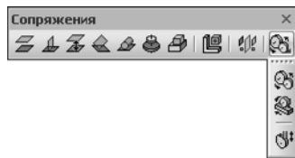
Рис. 2.11.13. Панель Сопряжения
