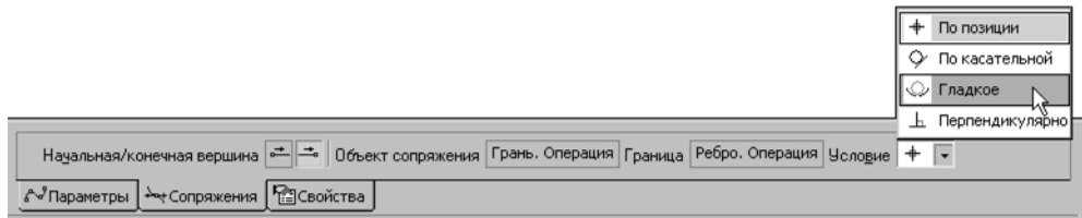
Рис. 2.5.23. Вкладка Сопряжения
