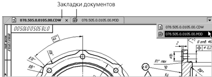
Рис. 1.2.8. Закладки документов
