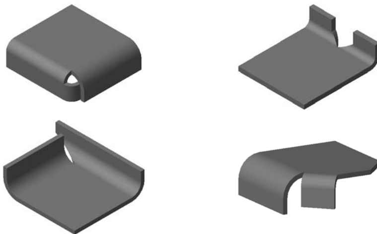
Рис. 2.4.73. Примеры смежных сгибов, замыкание угла между которыми невозможно
