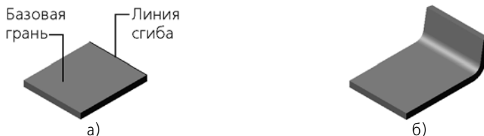
Рис. 2.4.35. Сгиб вдоль ребра: а) базовая грань и линия сгиба, б) результат построения
