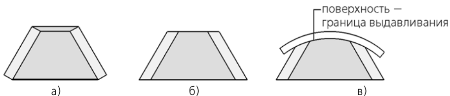
Рис. 2.4.15. Кромки оснований обечайки: а) перпендикулярно плоскости листа; б) совпадение с поверхностями оснований; в) совпадение с поверхностями оснований, способ До поверхности (для простой обечайки)
