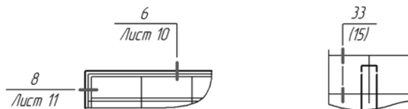
Рис. 3.3.114. Примеры обозначений узлов в сечении
