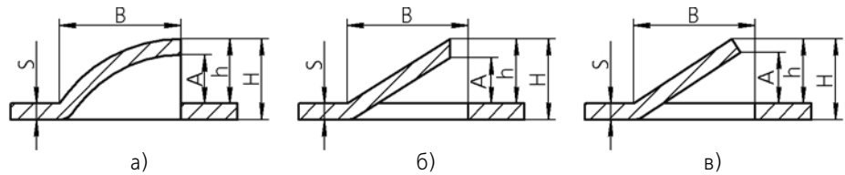
Рис. 2.4.116. Геометрические параметры жалюзи: а) вытянутых; б) подрезанных с торцем по направлению подрезки; в) подрезанных с торцем по нормали к толщине
