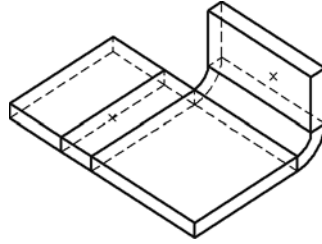
Рис. 2.4.86. Исходное состояние детали. Центры будущих отверстий (расположенные на невидимых гранях) обозначены «крестиками»
