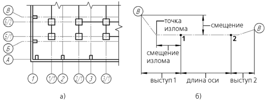
Рис. 3.3.123. Прямая координационная ось: а) пример использования, б) параметры оси
