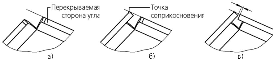
Рис. 2.4.68. Построение замыкания с перекрытием для тупого угла: а), б) определение положения перекрывающей стороны, в) определение положения перекрываемой стороны
