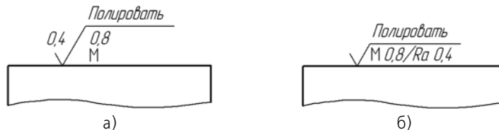
Рис. 3.3.52. Структура обозначения шероховатости: а) соответствующая предыдущей редакции ГОСТ 2.309–73, б) соответствующая изменению №3, 2003 в ГОСТ 2.309–73
