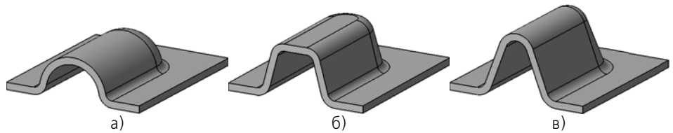
Рис. 2.4.111. Формы сечения буртиков
