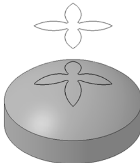
Рис. 2.5.52. Проекция эскиза на грань тела
