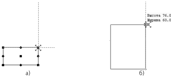
Рис. 3.5.4. Вспомогательные траектории: а) начальное положение характерной точки, б) «перетаскивание» характерной точки вдоль траектории
