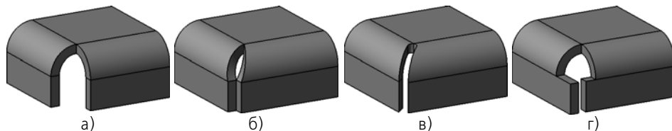
Рис. 2.4.57. Замыкание угла: а) исходное состояние детали, б), в), г) варианты замыкания угла
