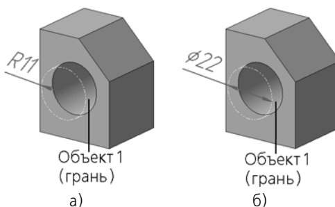
Рис. 2.9.12. Примеры простановки размеров к грани детали: а) радиального, б) диаметрального
