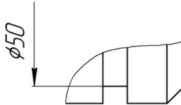
Рис. 3.3.16. Пример простановки размеров с обрывом
