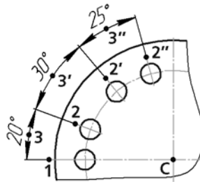
Рис. 3.3.42. Простановка цепи угловых размеров; способ задания сторон угла — по двум отрезкам
