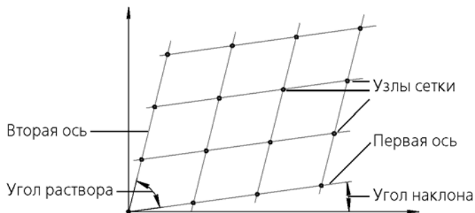
Рис. 3.5.14. Схема образования параллелограммной сетки
