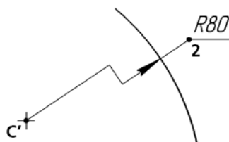
Рис. 3.3.31. Радиальный размер с надписью, размещенной на полке
