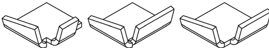
Рис. 2.4.59. Примеры несмежных сгибов
