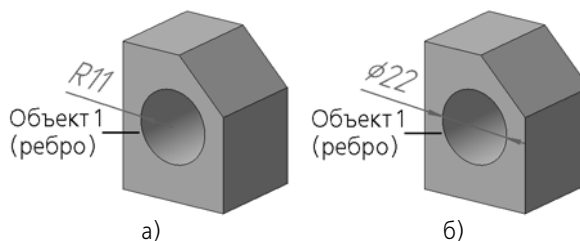
Рис. 2.9.11. Примеры простановки размеров к ребру детали: а) радиального, б) диаметрального
