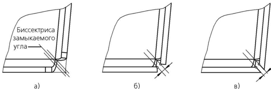
Рис. 2.4.64. Определение положения сторон угла при замыкании встык и плотном замыкании
