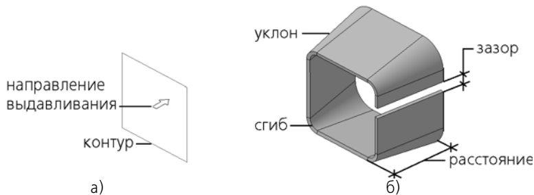
Рис. 2.4.20. Построение обечайки на основе замкнутого контура: а) эскиз; б) обечайка
