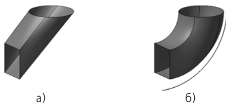
Рис. 2.6.10. Поверхность по сечениям: а) без осевой линии, б) с осевой линией
