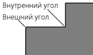
Рис. 2.4.81. Внутренний и внешний углы грани листового тела
