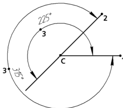
Рис. 3.3.37. Простановка размера на угол больше 180^\circ между отрезками
