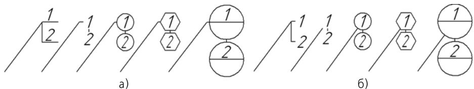
Рис. 3.3.67. Обозначения позиций различных форм: а) с полкой, б) без полки
