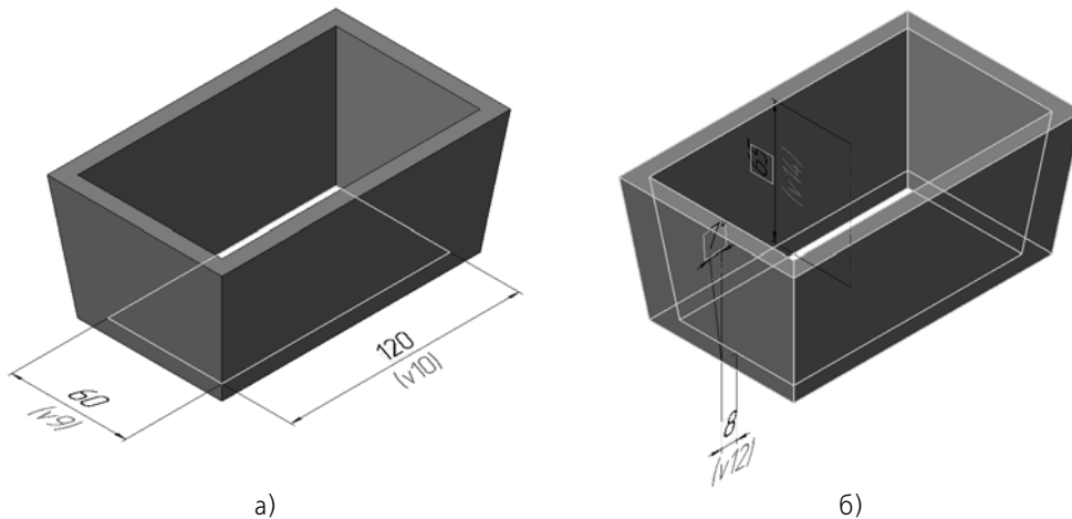
Рис. 2.9.4. Пример отображения размеров выделенного объекта: а) эскиза, б) элемента выдавливания
