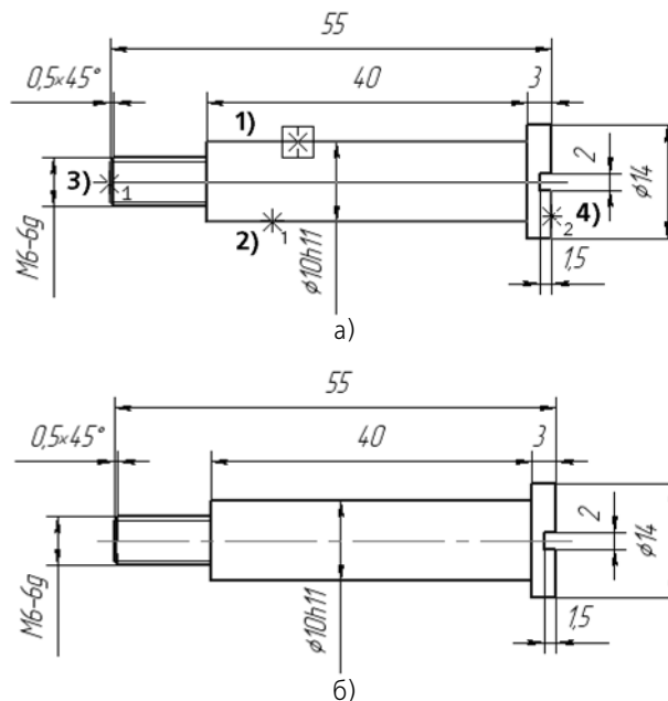
Рис. 3.3.88. Построение автоосевой на чертеже способом С указанием границы : а) указание объектов для построения автоосевой, б) построенная автоосевая
