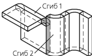
Рис. 2.4.30. Пример расположения сгибов, позволяющего применить освобождение угла: плоская кольцевая грань создаваемого Сгиба 1 частично совпадает с плоской прямоугольной гранью соседнего с ним Сгиба 2
