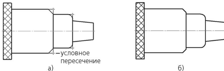
Рис. 3.2.98. Построение фаски/скругления: а) при включенном построении условного пересечения, б) при выключенном
