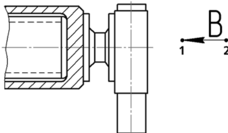
Рис. 3.3.70. Простановка стрелки направления взгляда
