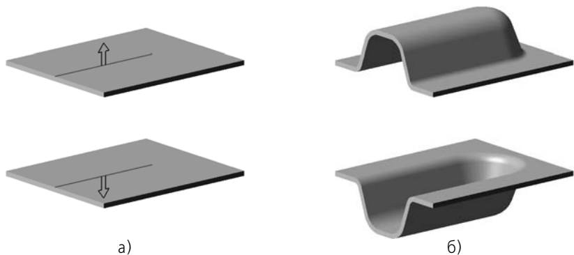
Рис. 2.4.106. Направление построения штамповочного элемента: а) выбор направления, б) результат построения
