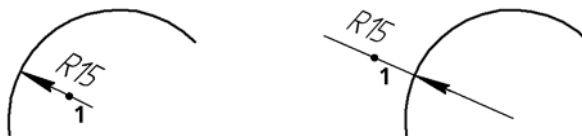
Рис. 3.3.25. Радиальный размер с автоматически размещенной надписью
