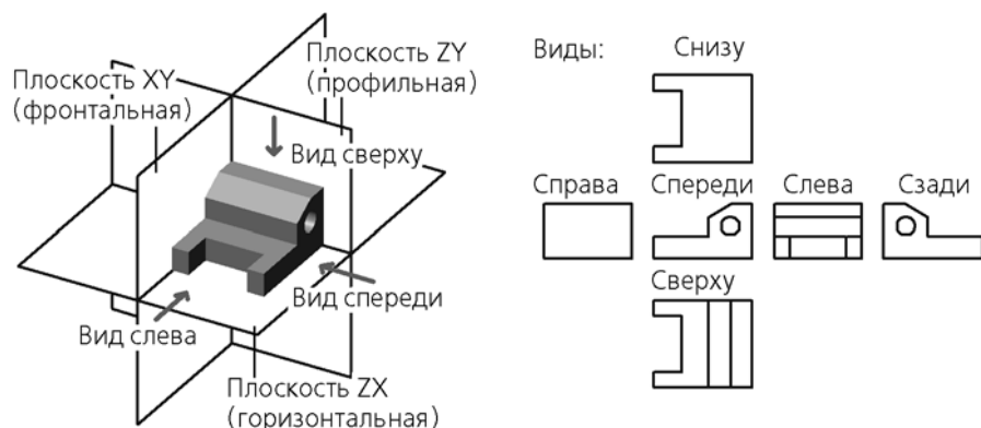
Рис. 2.2.1. Положение детали относительно координатных плоскостей
