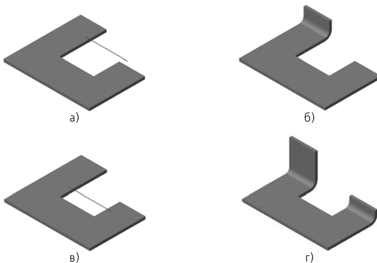
Рис. 2.4.48. Зависимость результата сгиба от положения линии сгиба: а), в) варианты положения линии сгиба, б), г) соответствующие результаты построения
