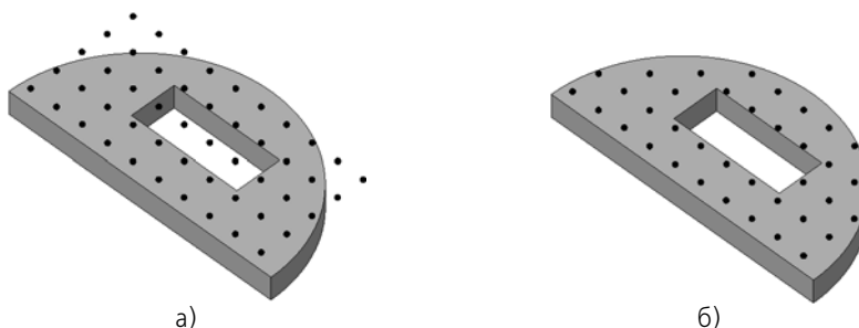
Рис. 2.5.9. Пример построения группы точек по поверхности: а) группа точек при отключенной опции Учитывать границы б) группа точек при включенной опции Учитывать границы
