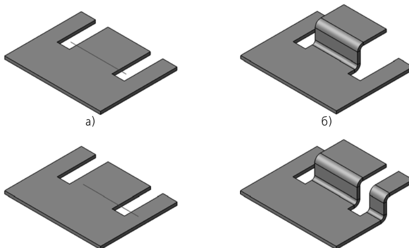
Рис. 2.4.52. Зависимость результата построения подсечки от положения линии сгиба: а), в) варианты положения линии сгиба, б), г) соответствующие результаты выполнения операции
