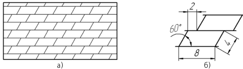
Рис. 11.1.37. Стиль штриховки Гранит: а) образец штриховки, б) размер и расположение элементов штриховки
