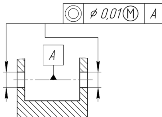
Рис. 3.3.77. Простановка допуска расположения поверхностей
