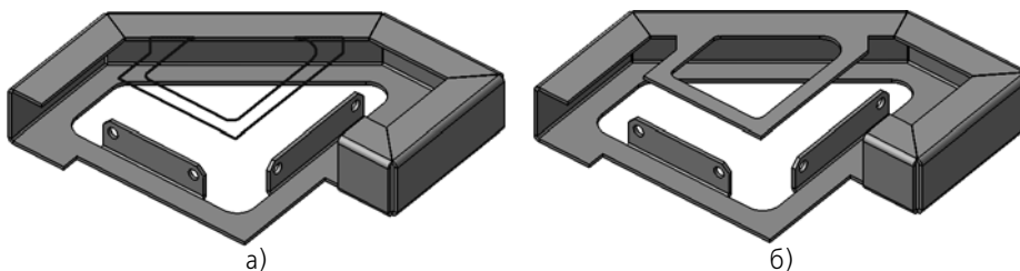
Рис. 2.4.85. Создание пластины: а) исходное состояние детали и эскиз пластины, б) результат операции
