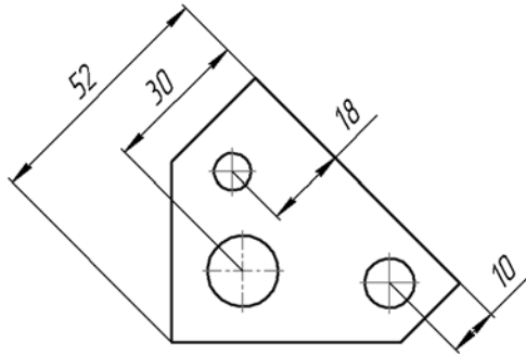
Рис. 3.3.17. Пример простановки размера между отрезком и точкой
