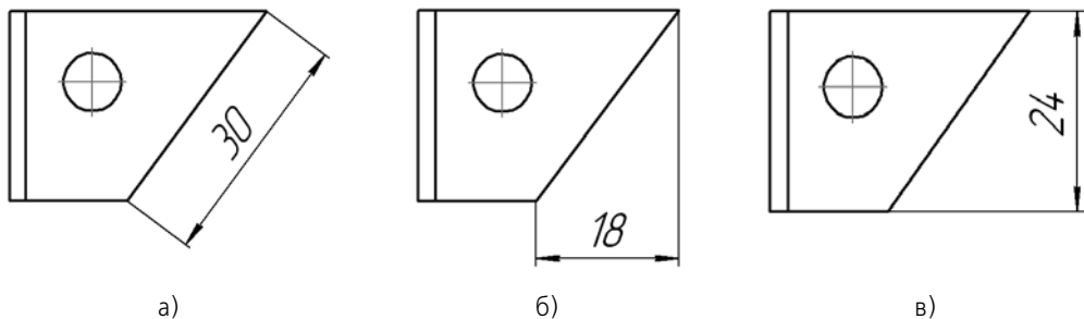
Рис. 3.3.14. Ориентация линейного размера: а) параллельный объекту, б) горизонтальный, в) вертикальный
