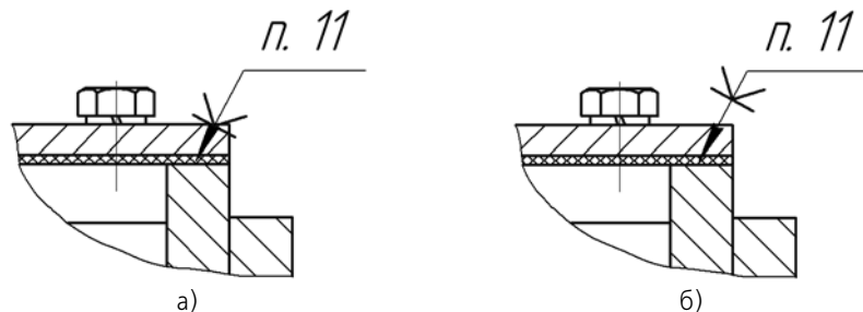
Рис. 3.3.61. Изменение положения значка на линии-выноске: а) положение значка по умолчанию, б) значок перемещен вверх по линии-выноске
