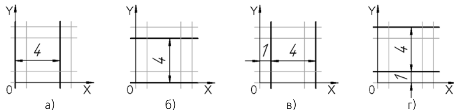
Рис. 11.1.26. Группы линий, составляющие штриховку Фарфор: а) группа 1, б) группа 2, в) группа 3, г) группа 4
