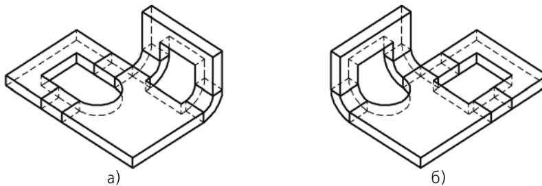
Рис. 2.4.92. Вырезы, построенные способом На глубину : а) вид детали сразу после создания вырезов, б) результат изменения состояния сгибов
