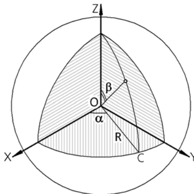
Рис. 2.5.13. Построение точки по сферическим координатам; XYZ – система координат точки
