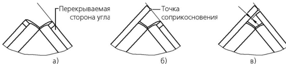
Рис. 2.4.67. Построение замыкания с перекрытием для острого угла: а), б) определение положения перекрывающей стороны, в) определение положения перекрываемой стороны
