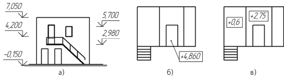
Рис. 3.3.47. Размер высоты: а) для вида спереди или разреза, б) для вида сверху с линией-выносной, в) для вида сверху непосредственно на изображении
