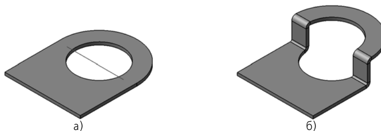
Рис. 2.4.55. Подсечка в детали с отверстием: а) положение линии сгиба, б) результат построения
