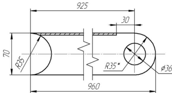
Рис. 3.6.16. Пример разрыва изображения
