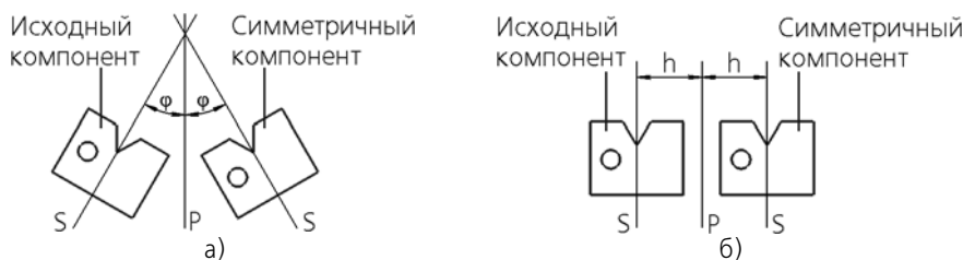
Рис. 2.11.11. Размещение компонента с использованием его плоскости симметрии: а) плоскость симметрии компонента не параллельна плоскости симметрии операции; б) плоскость симметрии компонента параллельна плоскости симметрии операции
