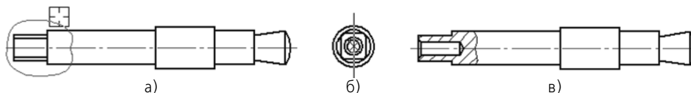
Рис. 3.7.10. Построение местного разреза: а) указание контура, ограничивающего разрез, б) указание положения секущей плоскости, в) результат выполнения команды
