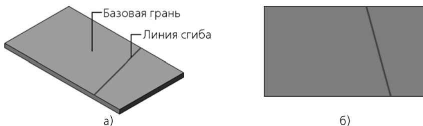
Рис. 2.4.56. Исходный элемент подсечки: а) изометрическая проекция, б) проекция исходного элемента на базовую грань
