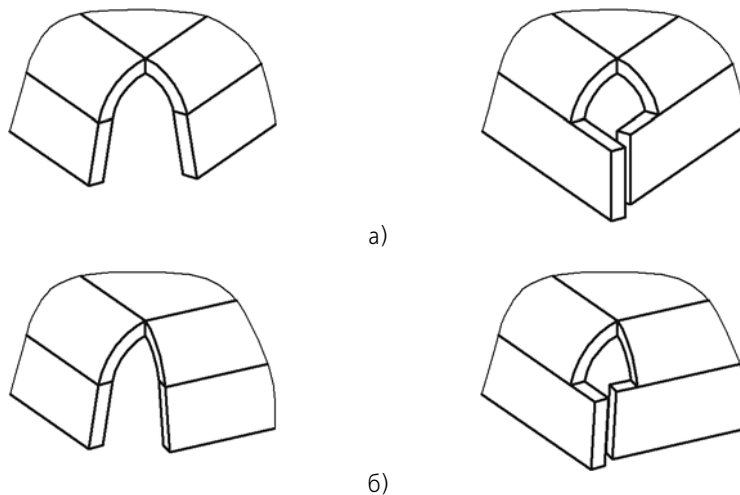
Рис. 2.4.66. Замыкание с перекрытием (исходное состояние детали и результат операции): а) замыкаемый угол острый, б) замыкаемый угол тупой
