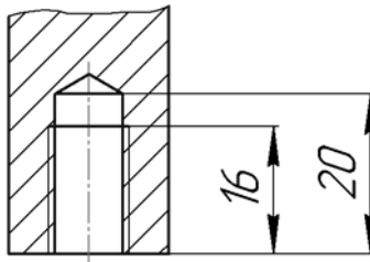
Рис. 3.3.18. Простановка линейных размеров от общей базы
