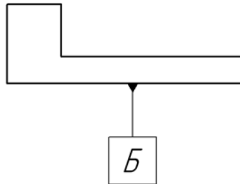
Рис. 3.3.75. Пример простановки обозначения базы
