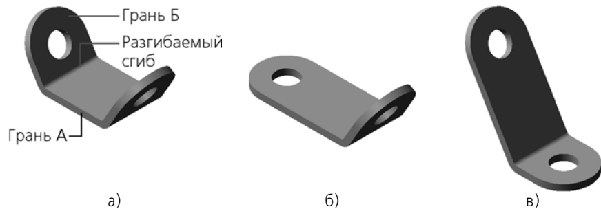
Рис. 2.4.93. Зависимость результата разгибания от выбора плоскости разгибания: а) исходное состояние детали, б) плоскость разгибания – грань А, в) плоскость разгибания – грань Б
