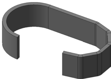
Рис. 2.4.23. Пример обечайки с сегментированным и несегментированным участками
