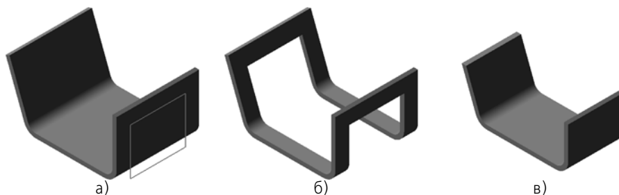
Рис. 2.4.89. Результат построения выреза в листовом теле: а) исходное состояние детали и эскиз выреза, б) вырез вычитанием, в) вырез пересечением
