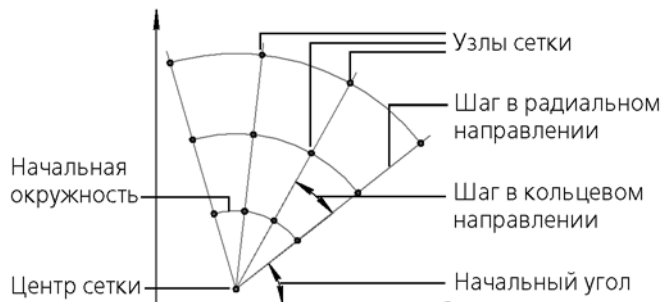
Рис. 3.5.16. Схема образования концентрической сетки
