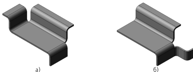
Рис. 2.4.77. Сгиб вдоль цепочки ребер: а) соединенных вершиной, б) соединенных сгибом
