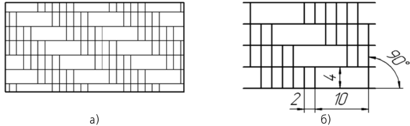
Рис. 11.1.36. Стиль штриховки Соли: а) образец штриховки, б) размер и расположение элементов штриховки
