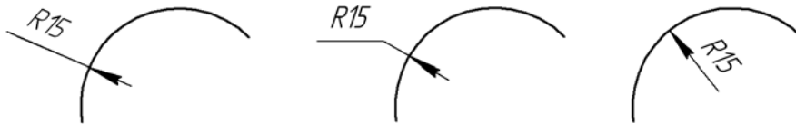
Рис. 3.3.27. Радиальный размер не от центра
