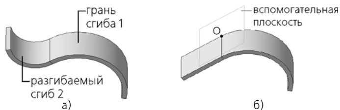
Рис. 2.4.94. Разгибание листового тела: а) исходное состояние детали, б) результат разгибания сгиба 2 (при указании грани сгиба 1)
