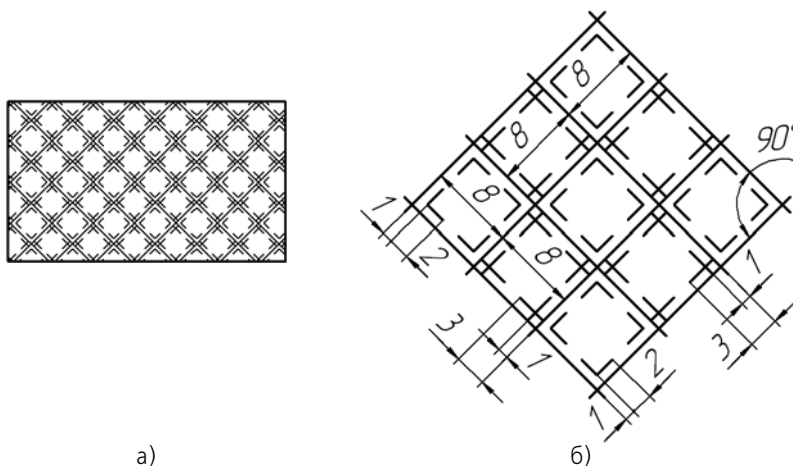
Рис. 11.1.28. Стиль штриховки Термопласт: а) образец штриховки, б) размер и расположение элементов штриховки
