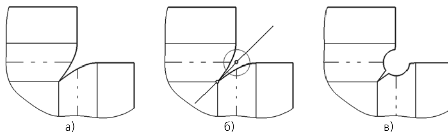
Рис. 2.4.60. Построение замыкания угла с круговой обработкой: а) построение замыкания угла с обработкой Стык по кромке ; б) размещение отверстия; в) результат построения
