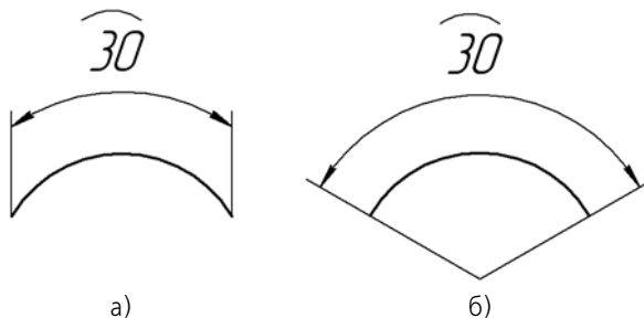
Рис. 3.3.21. Размер дуги: а) с параллельными выносными линиями, б) с выносными линиями от центра
