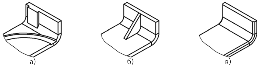
Рис. 2.4.99. Примеры формообразующих и конструктивных элементов, делающих невозможным разгибание сгиба: а) приклеенный и вырезанный элементы, б) ребро жесткости, в) фаска
