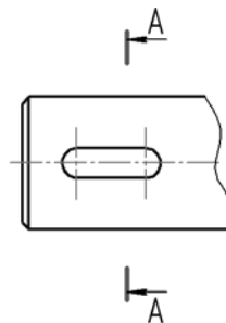
Рис. 3.3.72. Простановка линии разреза
