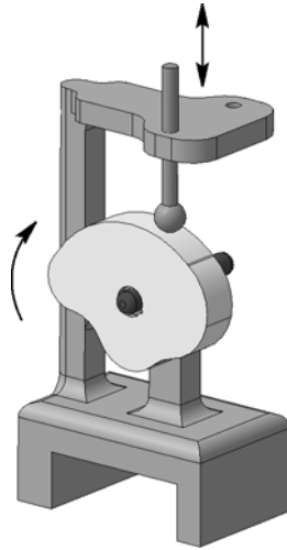
Рис. 2.11.18. Пример применения сопряжения Кулачок – толкатель
