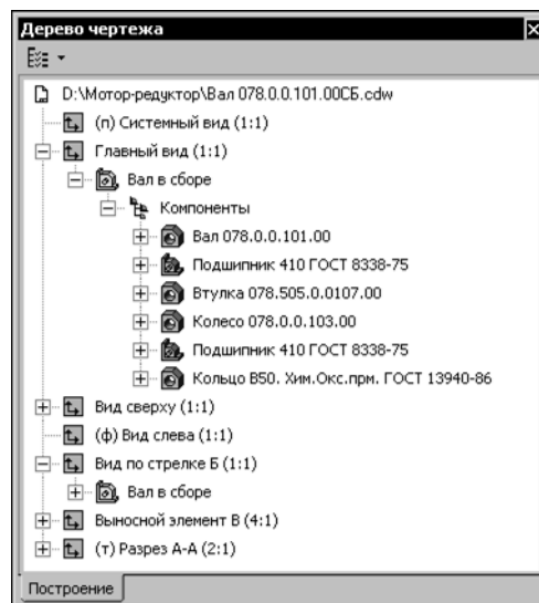
Рис. 3.6.8. Дерево чертежа
