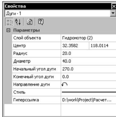
Рис. 3.5.5. Свойства дуги
