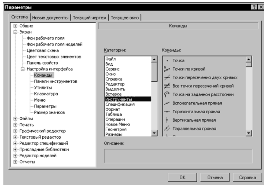
Рис. 9.4.1. Диалог Команды
