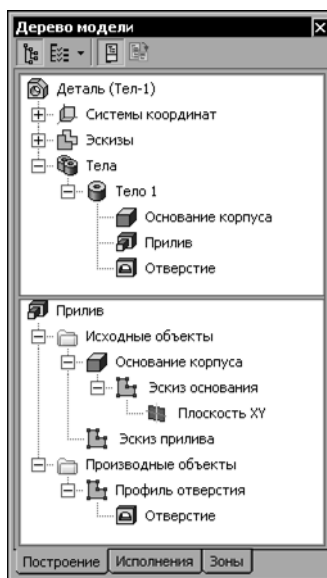
Рис. 2.1.8. Просмотр иерархии
