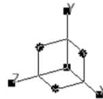
Рис. 2.8.6. Фантом ЛСК
