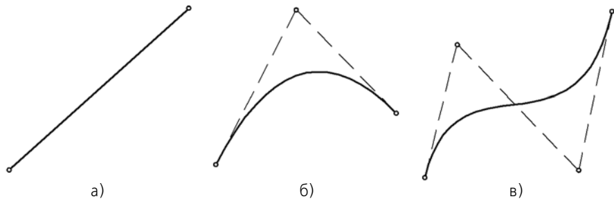
Рис. 3. Частные случаи сплайновых кривых: а) линейная кривая (количество полюсов – 2, порядок – 2, степень полинома – 1), б) коническая кривая (количество полюсов – 3, порядок – 3, степень полинома – 2), в) кубическая кривая (количество полюсов – 4, порядок – 4, степень полинома – 3)
