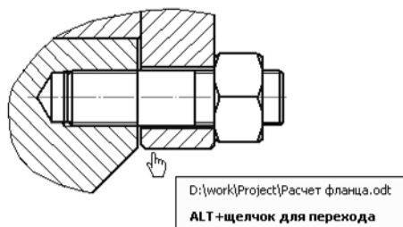
Рис. 10.2.1. Отображение гиперссылки
