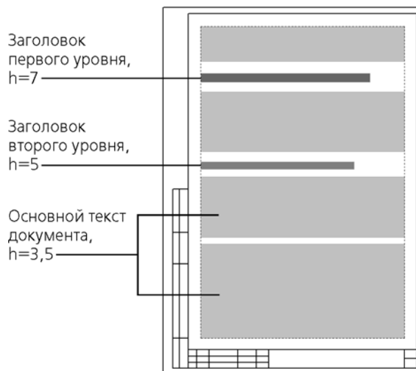
Рис. 11.1.44. Макет страницы
