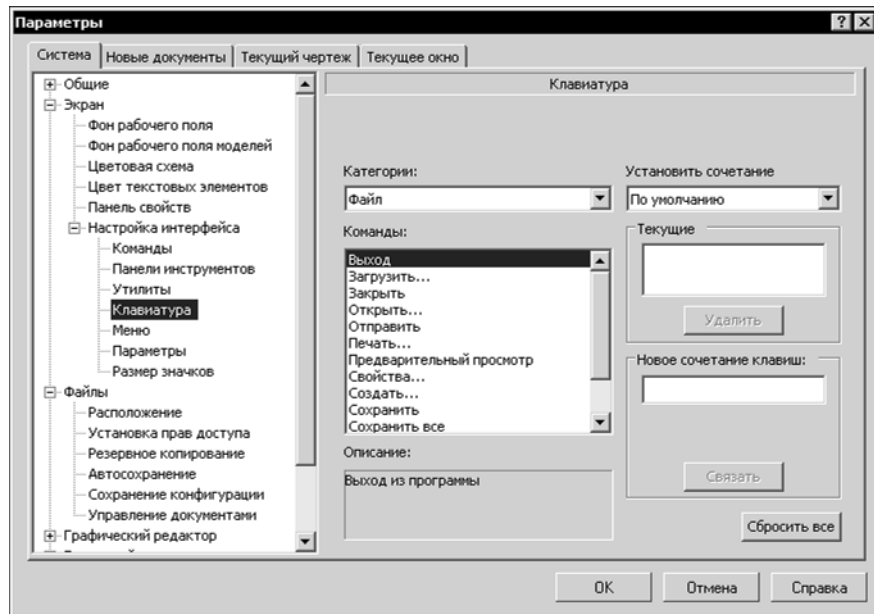
Рис. 9.4.3. Диалог Клавиатура
