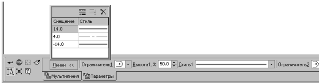
Рис. 3.2.77. Панель Линии
