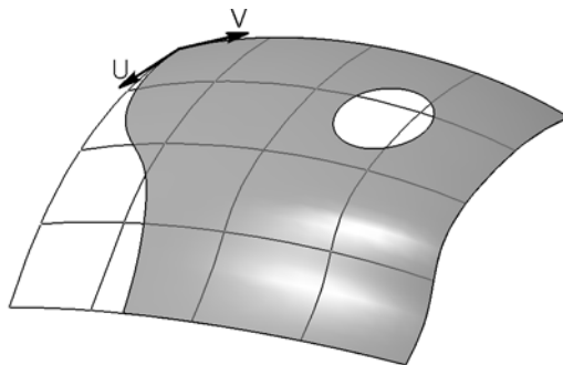
Рис. 2. Пример изопараметрической сети
