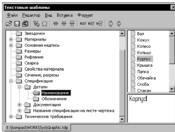
Рис. 6.2.13. Текстовые шаблоны
