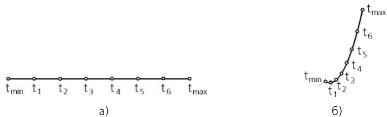
Рис. 1. Полукубическая парабола (парабола Нейля):
