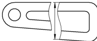
Рис. 3.6.19. Длина разрыва
