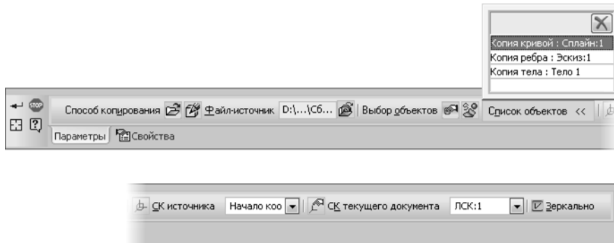
Рис. 2.8.17. Вкладка Параметры
