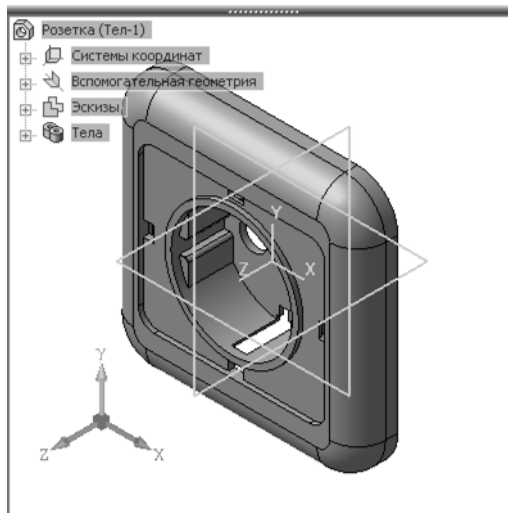
Рис. 2.8.18. Окно модели-источника
