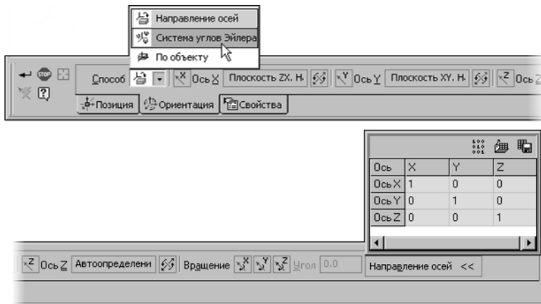
Рис. 2.8.9. Вкладка Ориентация
