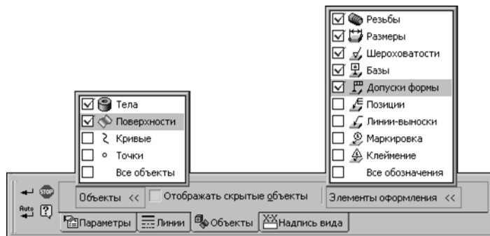
Рис. 3.7.6. Вкладка Объекты
