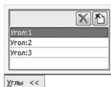
Рис. 2.4.71. Панель Углы
