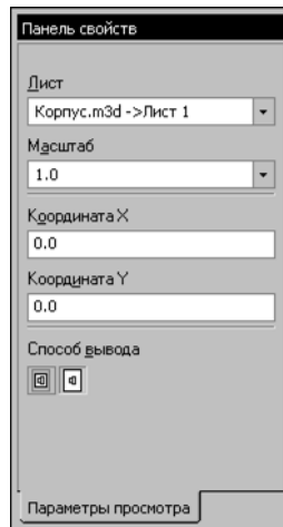
Рис. 8.3.2. Панель свойств
