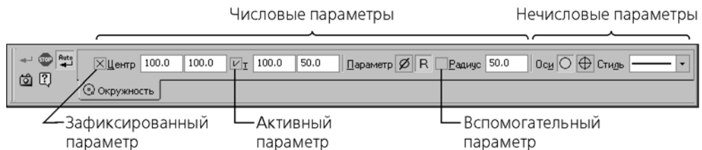
Рис. 1.4.5. Параметры окружности
