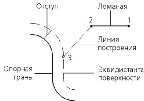
Рис. 2.5.22. Определение положения вершины путем задания ее смещения от опорной грани
