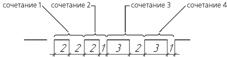
Рис. 11.1.30. Сочетания штрихов и промежутков в прерывистых линиях штриховки Термопласт
