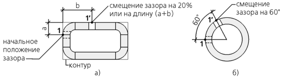
Рис. 2.4.19. Смещение зазора: а) по параметру U или по длине; б) по центральному углу
