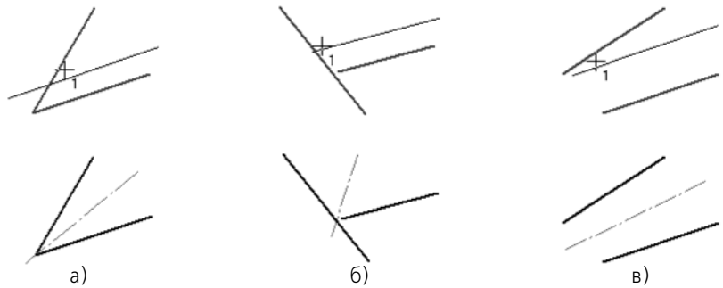
Рис. 3.3.82. Примеры построения автоосевой
