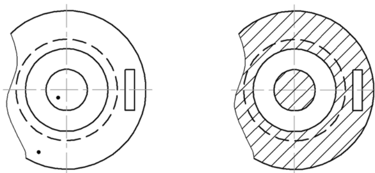
Рис. 3.2.84. Построение штриховки: а) точки внутри областей, указанные для построения, б) полученная штриховка
