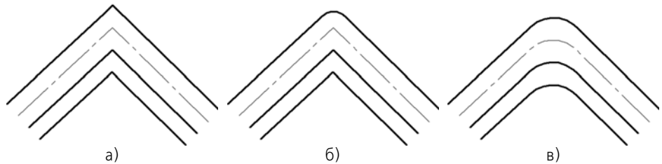
Рис. 3.2.80. Способы обхода угла в вершине базовой линии: а) обход срезом, б) обход скруглением, в) обход скруглением с одинаковым радиусом
