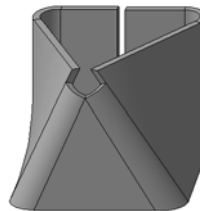
Рис. 2.4.25. Пример освобождения угла при пересечении сгибов линейчатой обечайки
