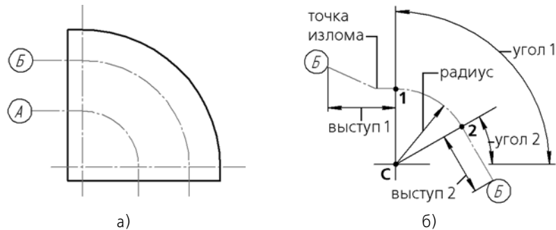
Рис. 3.3.130. Дуговая координационная ось: а) пример использования, б) параметры оси
