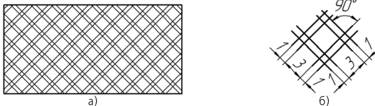
Рис. 11.1.35. Стиль штриховки Изоляционный слой : а) образец штриховки, б) размер и расположение элементов штриховки
