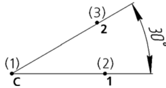
Рис. 3.3.35. Пример простановки углового размера по трем точкам
