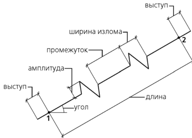
Рис. 3.3.98. Параметры линии с изломами
