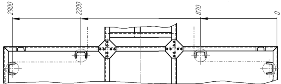
Рис. 3.3.20. Простановка линейных размеров с общей размерной линией
