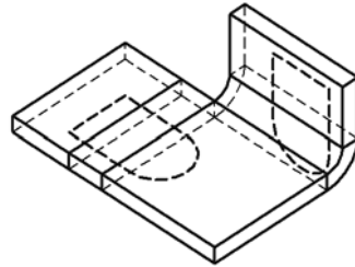
Рис. 2.4.90. Исходное состояние детали. Эскизы вырезов (расположенные на невидимых гранях) показаны основной штриховой линией
