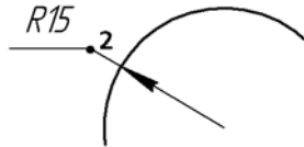
Рис. 3.3.26. Радиальный размер на полке
