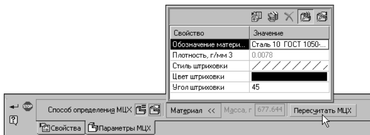
Рис. 2.14.14. Задание плотности модели
