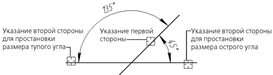
Рис. 3.3.36. Автоопределение типа углового размера
