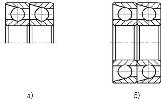
Рис. 3.5.23. Преобразование симметрии: а) исходное изображение, б) результат выполнения команды
