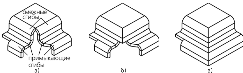
Рис. 2.4.62. Замыкание сгиба: а) исходное состояние детали, б) замыкание без продолжения, в) замыкание с продолжением
