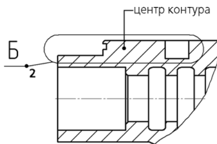
Рис. 3.3.74. Обозначение положения выносного элемента
