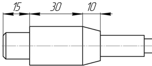
Рис. 3.3.19. Простановка цепи линейных размеров
