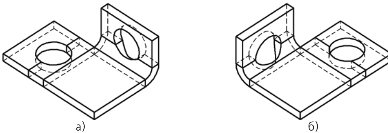
Рис. 2.4.87. Отверстия, построенные способом По толщине : а) вид детали сразу после создания отверстий, б) результат изменения состояния сгибов
