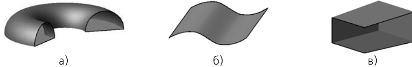
Рис. 2.6.36. Примеры открытых ребер (выделены черным цветом): а) поверхность вращения, б) поверхность выдавливания, в) тело с нарушенной целостностью
