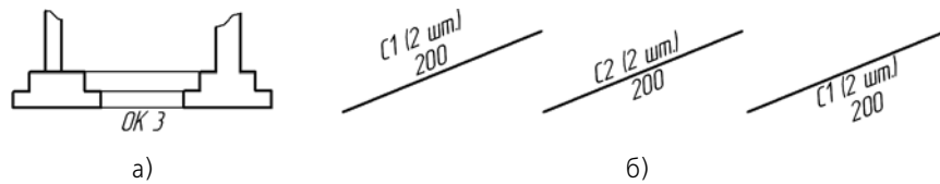
Рис. 3.3.109. Марка/позиционное обозначение на линии: а) пример использования, б) варианты размещения текста
