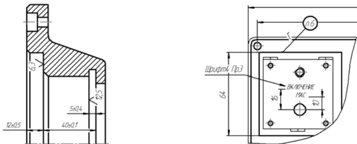
Рис. 3.5.30. Усечение объектов по двум точкам
