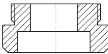
Рис. 3.2.85. Штриховка, состоящая из нескольких областей
