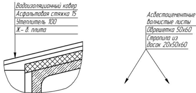
Рис. 3.3.121. Примеры выносной надписи
