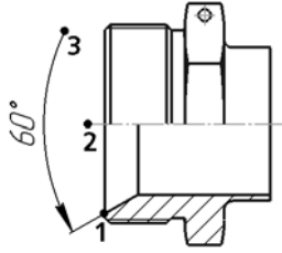
Рис. 3.3.44. Простановка углового размера с обрывом; способ задания сторон угла — по двум отрезкам
