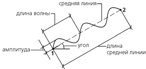
Рис. 3.3.91. Параметры волнистой линии
