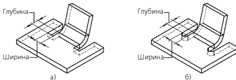
Рис. 2.4.44. Освобождение сгиба: а) прямоугольное, б) скругленное
