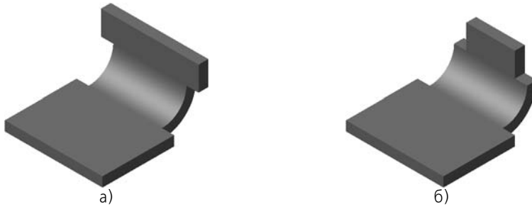
Рис. 2.4.42. Изменение ширины продолжения сгиба: а) увеличение, б) уменьшение
