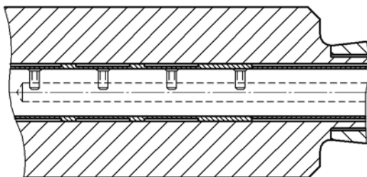
Рис. 3.5.11. Пример копирования по кривой
