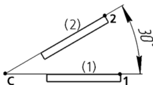
Рис. 3.3.33. Пример простановки углового размера по двум отрезкам
