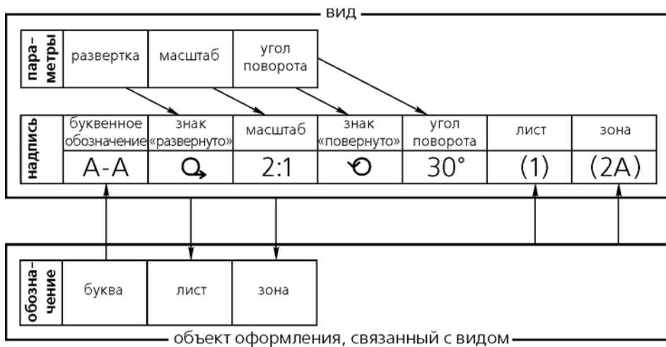
Рис. 3.6.10. Схема связей между надписью вида и обозначением линии разреза (для машиностроения), связанного с этим видом
