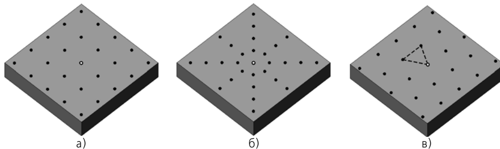
Рис. 2.5.8. Группа точек, построенная способом По сетке вокруг заданной точки : а) прямоугольная сетка; б) концентрическая сетка; в) гексагональная сетка
