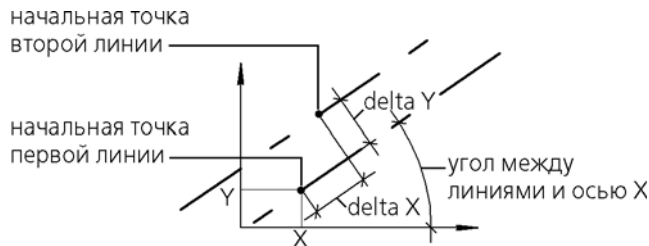
Рис. 11.1.23. Параметры группы линий штриховки
