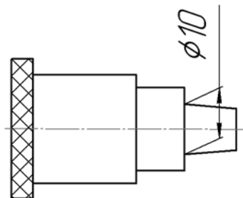
Рис. 3.3.15. Пример простановки размера с наклонными выносными линиями
