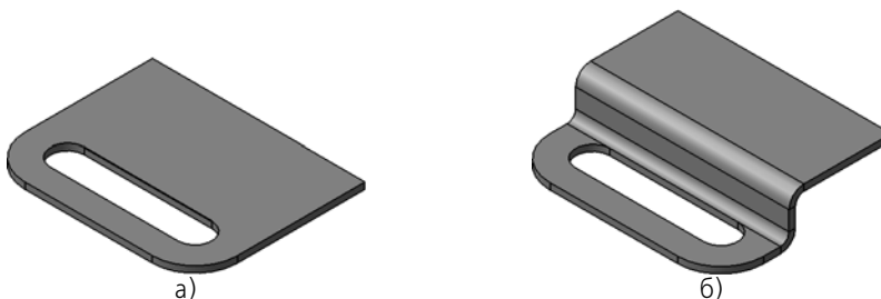
Рис. 2.4.54. Использование ребра в качестве линии сгиба подсечки: а) расположение ребра, б) результат построения
