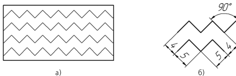
Рис. 11.1.38. Стиль штриховки Смола: а) образец штриховки, б) размер и расположение элементов штриховки
