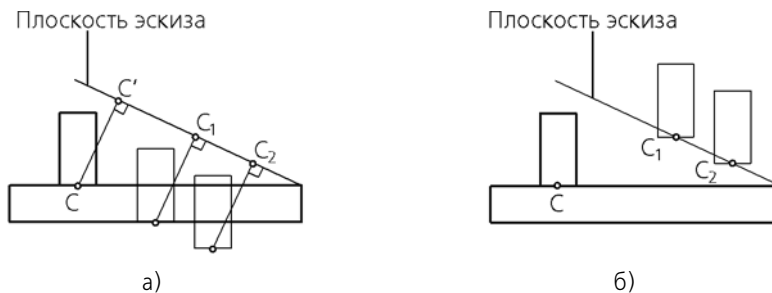
Рис. 2.7.35. Задание позиций экземпляров массива: а) при включенной опции Проецировать ; б) при отключенной опции Проецировать
