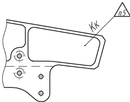
Рис. 3.3.62. Простановка обозначения клеймения
