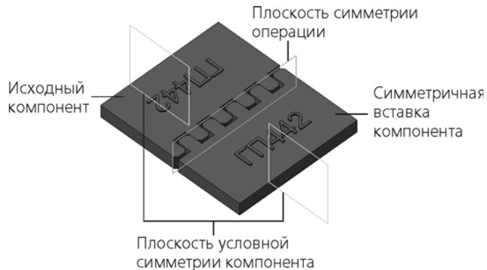
Рис. 2.11.7. Симметричная вставка компонента, обладающего условной симметрией
