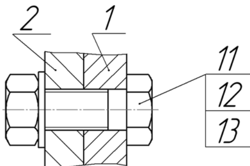
Рис. 3.3.65. Простановка позиционных линий-выносок
