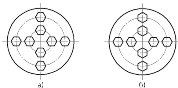
Рис. 3.5.18. Копирование по концентрической сетке: а) без доворота до радиального направления, б) с доворотом до радиального направления
