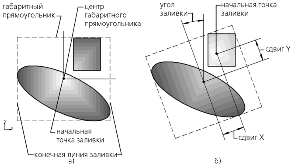
Рис. 3.2.89. Параметры заливки при построении: а) при отсутствии сдвига и угла наклона, б) после задания сдвига и угла наклона
