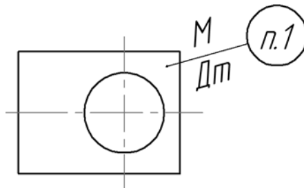
Рис. 3.3.64. Простановка обозначения маркировки
