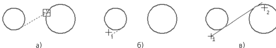
Рис. 3.2.60. Построение первого отрезка линии касательно к двум объектам: а) указание объектов, б) указание начальной точки отрезка, в) указание конечной точки отрезка
