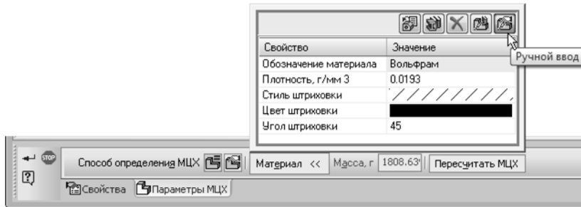
Рис. 2.14.7. Расчет МЦХ по плотности; панель Материал
