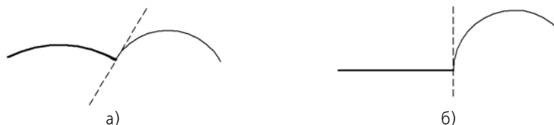
Рис. 3.2.71. Дуга по нормали: а) к дуге, б) к отрезку
