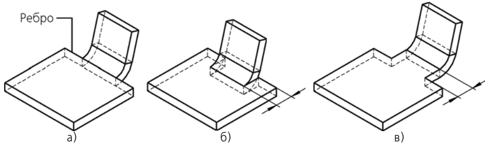
Рис. 2.4.41. Смещение сгиба: а) нулевое, б) внутрь, в) наружу
