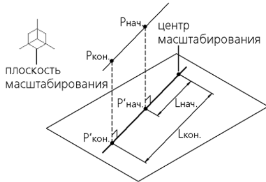
Рис. 2.6.53. Перемещение полюса при масштабировании в плоскости, плоскостью масштабирования является плоскость XY
