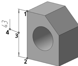
Рис. 2.9.6. Линейный размер на полке
